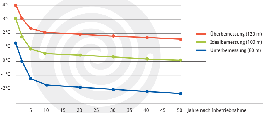
Temperaturentwicklung im Untergrund – Szenarien bei Über- oder Unterbemessung
